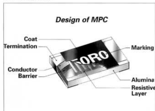
Ontwerp van de MPC 01 precisie-chipweerstande.
