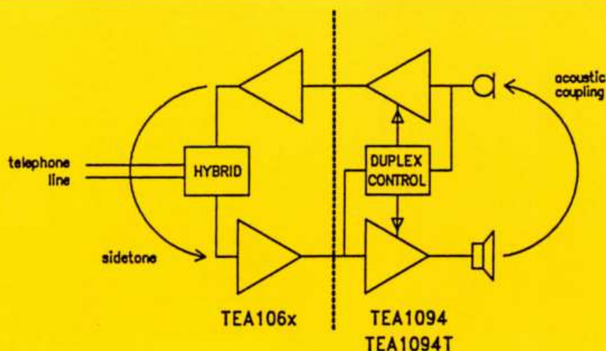
Principe-opbouw van een 'hands free'-telefoontoestel.
